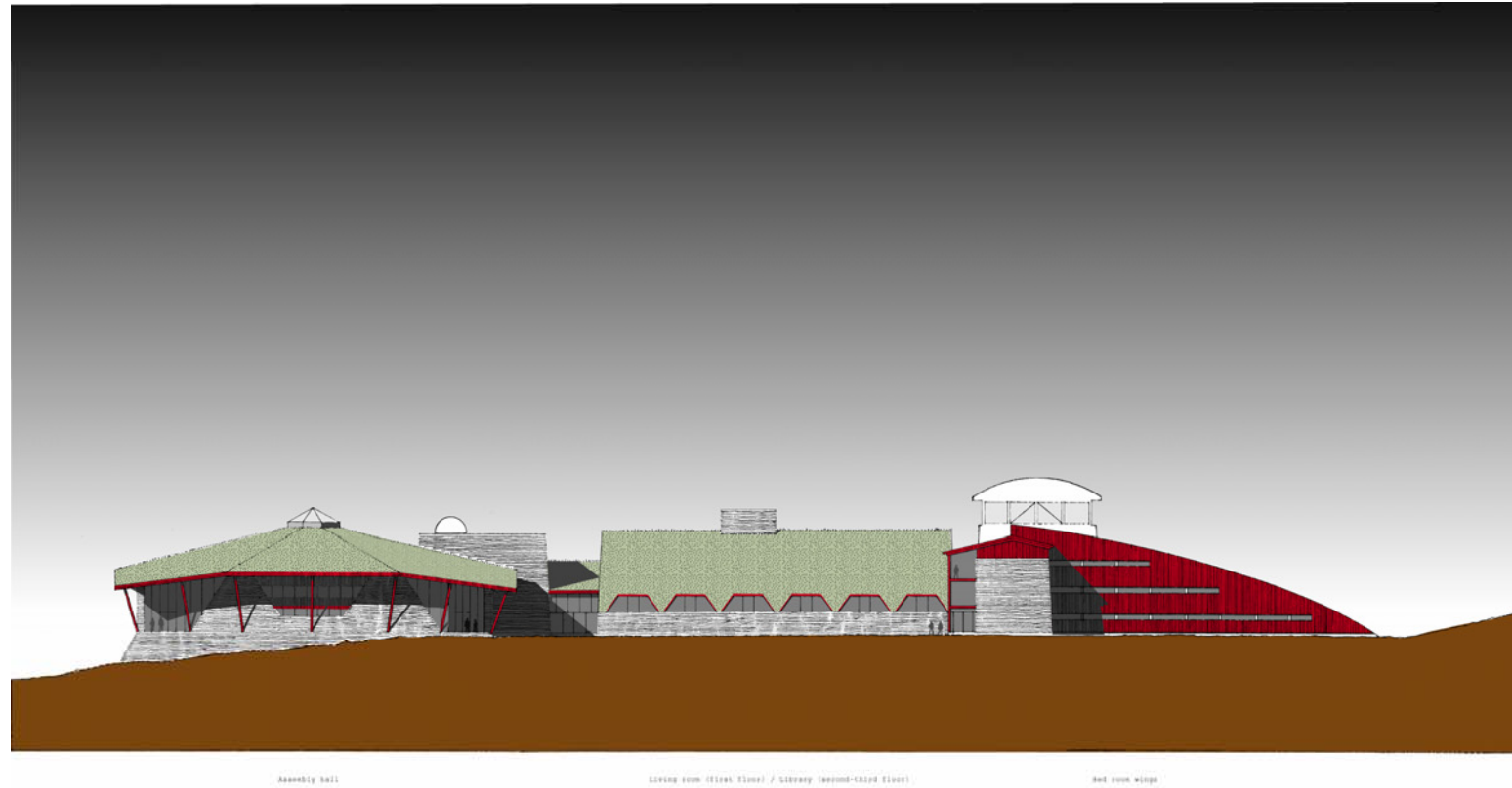
Fasade mot nord Målestokk 1:750
