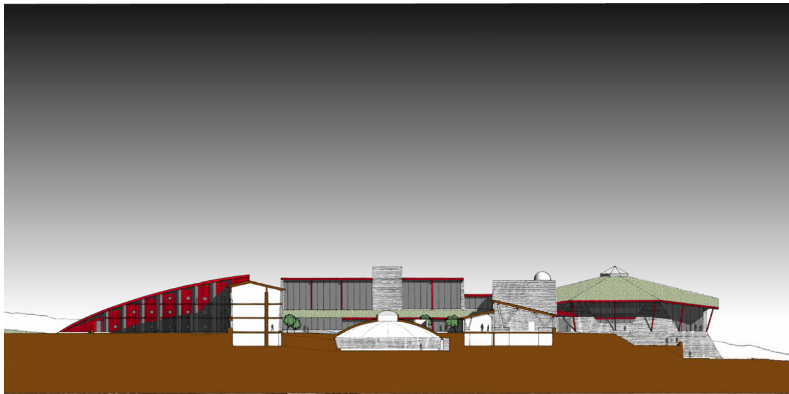
Fasade/snitt vest-øst Målestokk 1:750
